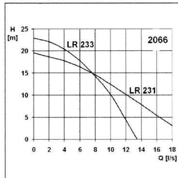
max. zulässiger Pumpendruck 4 bar *Edelstahl-Laufrad auf Anfrage
