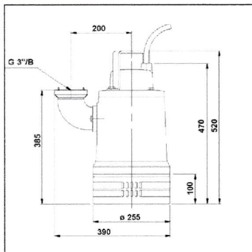
Sieböffnung 7 x 21 mm (alle Maße in mm)
